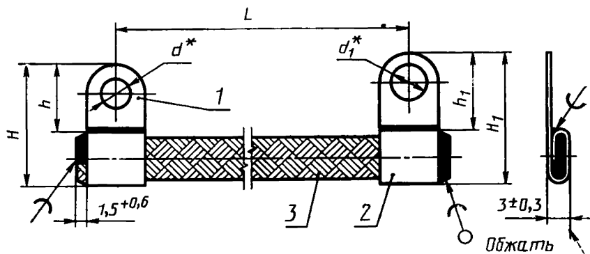
Перемычка типа Г
