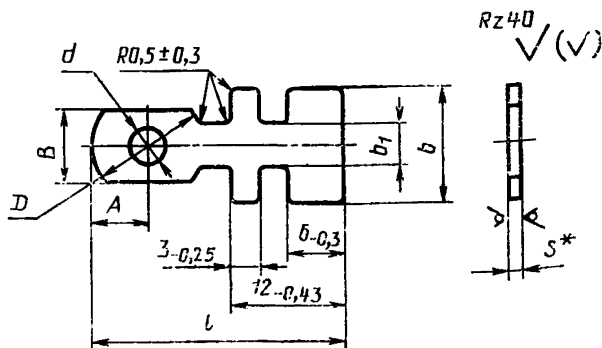
Наконечник типа Б
