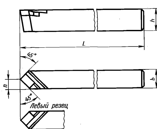
Исполнение 2
