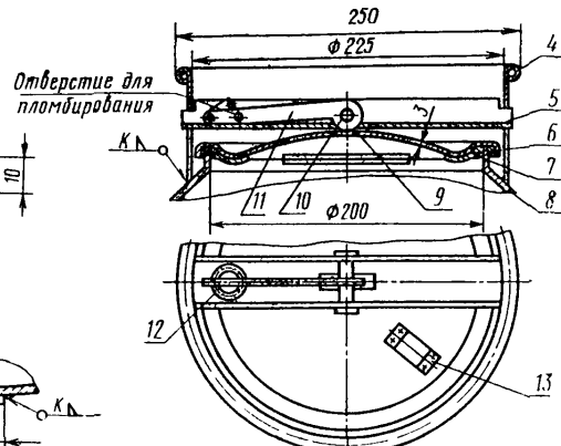
Исполнение Б
