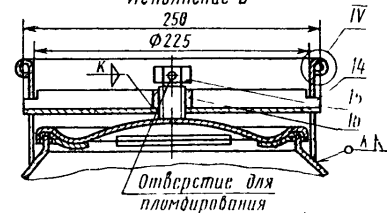
Исполнение Б
