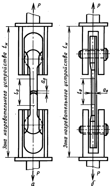
Схема испытаний сегментных образцов с головками
