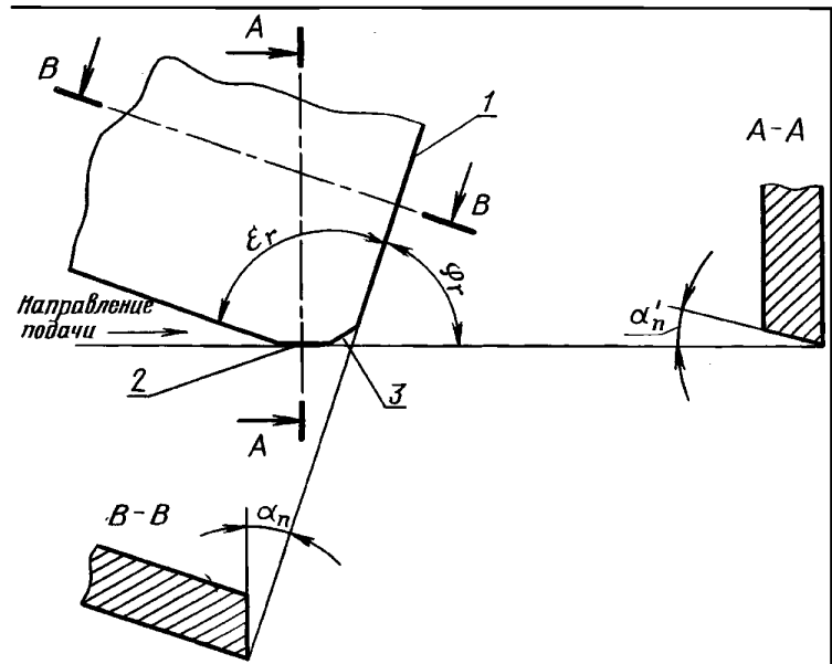
T — главная режущая кромка; 2 — зачистная режущая фаска; 3 — переходная фаска Черт. 4
