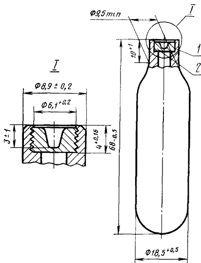
1—корпус; 2—пробка
