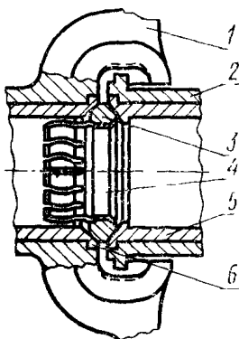
Соединение гаек с помощью двух штуцеров
