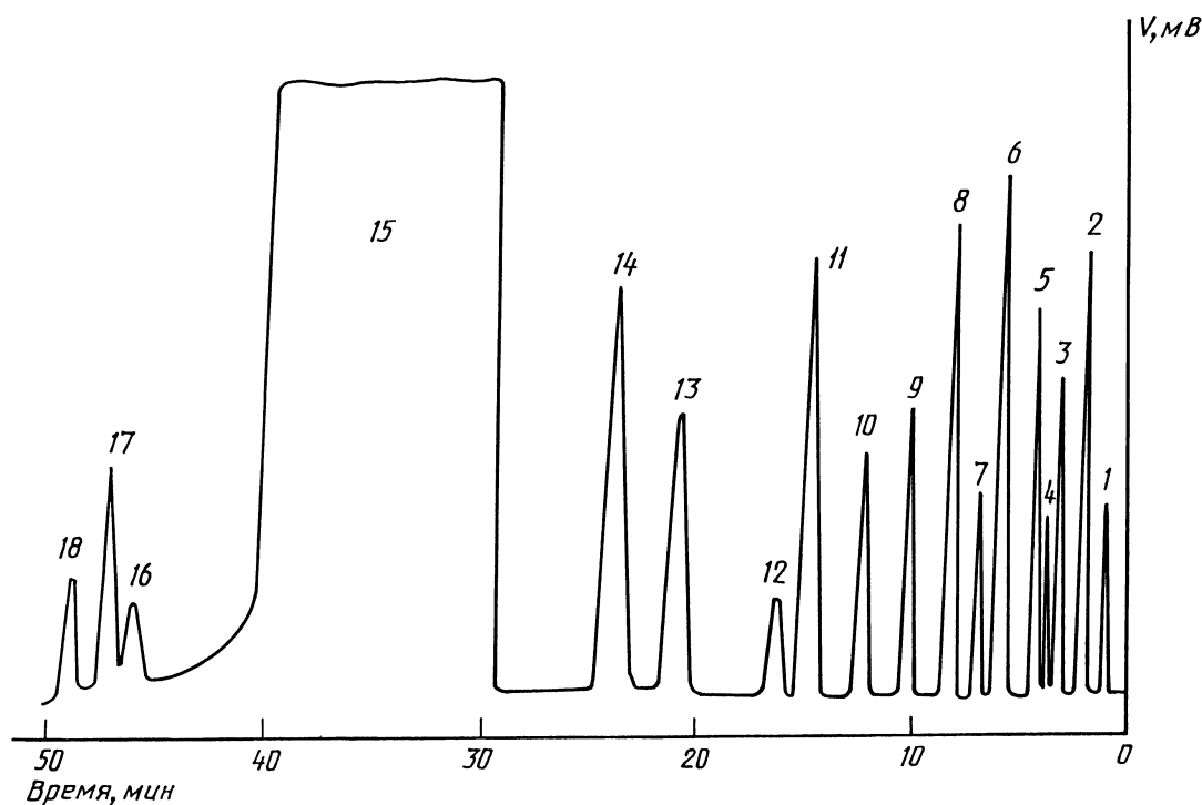
Типовая хроматограмма 1,2-дихлорэтана
