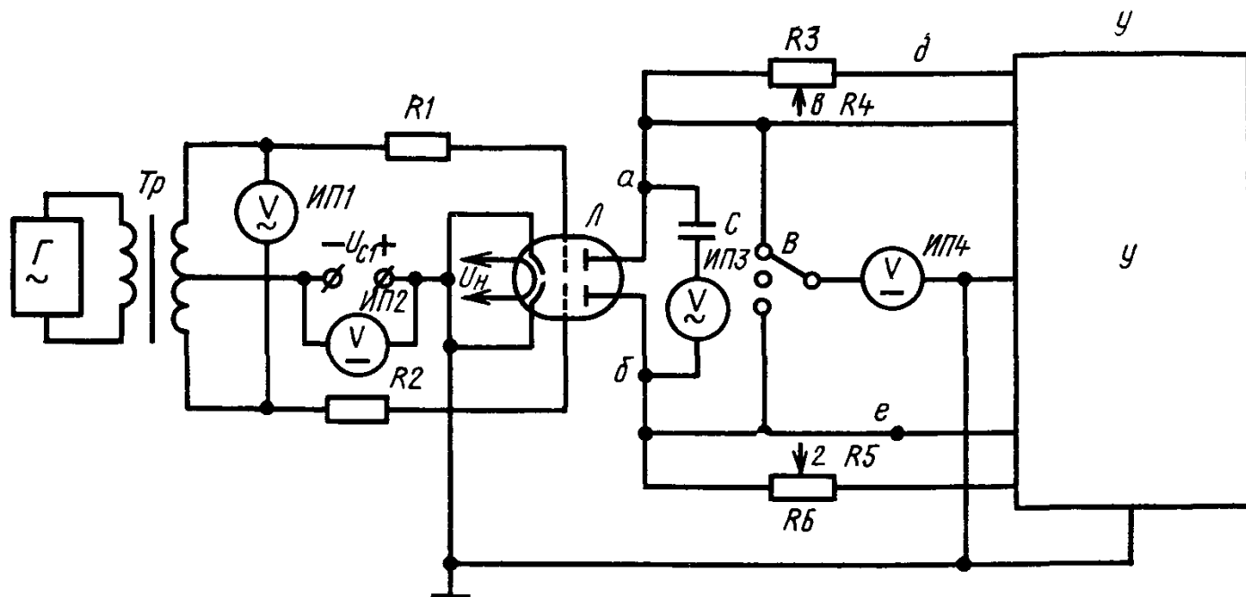
R1, R2, R3, R6 —резисторы; C —конденсатор; Л —испытуемая лампа; Tr —трансформатор; ИП1, ИП3 —вольтметры переменного тока; ИП2, ИП4 —вольтметры постоянного тока; B —переключатель; Г —генератор синусоидального напряжения, У —источник питания анодов, непосредственно стабилизирующий напряжения анода.
