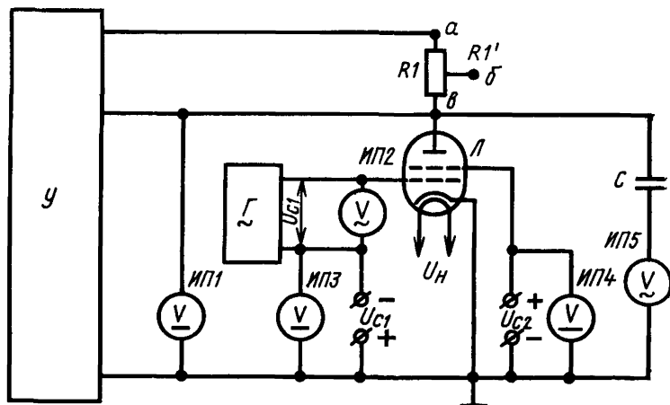
R1 —резистор; C —конденсатор; Л —испытуемая лампа; ИП1, ИП3, ИП4 —вольтметры постоянного тока; ИП2, ИП5 —вольтметры переменного тока; Г —генератор синусоидального напряжения; У —источник питания анода, непосредственно стабилизирующий напряжение анода.
