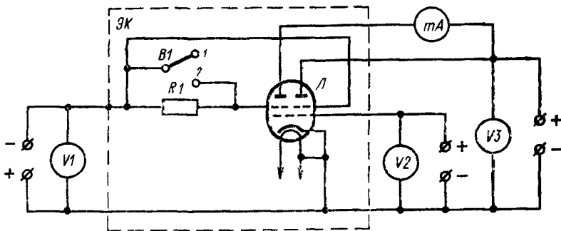
V1 , V2 , V3 —вольтметры постоянного тока; mA —миллиамперметр постоянного тока; B1 —выключатель; R1 —резистор; L —испытываемая лампа; ЭК —экранирующая камера.
