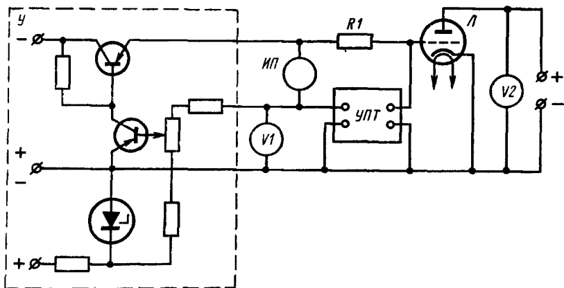
Y — одна из возможных схем транзисторного стабилизатора напряжения; V1 , V2 — вольтметры постоянного тока; ИП — измерительный прибор; УПТ — усилитель постоянного тока; R1 — резистор; Л — испытываемая лампа.
