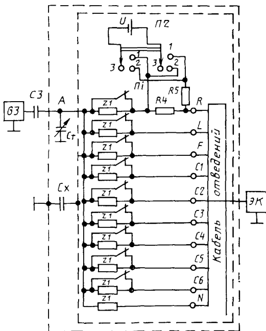
Схема определения коэффициента ослабления синфазных сигналов
