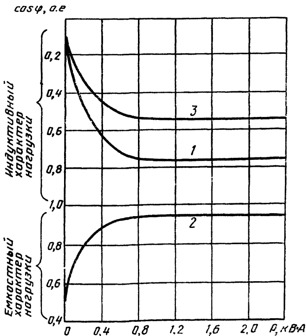
Пределы 1—3 значений коэффициента мощности приемников
