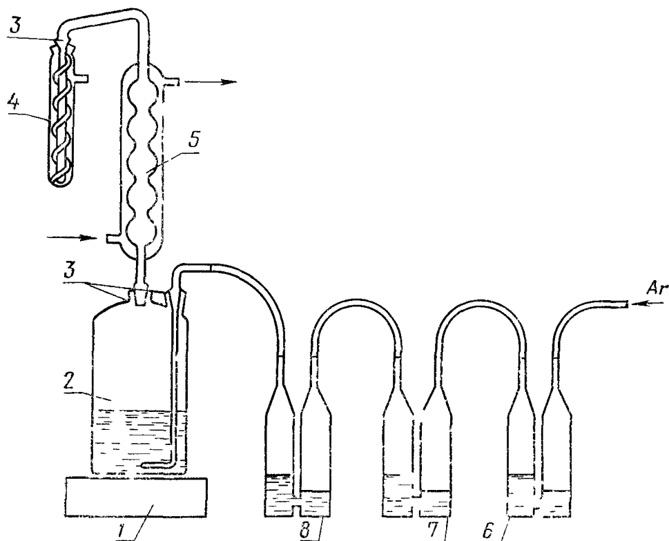
1—электроплитка, 2—сосуд реакционный с восстановительной смесью, 3—шлифы, 4—приемник с щелочным раствором гидроксиламина и трилона Б (спиральная кварцевая насадка приваренная к наружной стороне выходной трубки обратного холодильника), 5—обратный холодильник 6, 7—барботер с 25 % ным раствором пирогаллола в 25 % ном растворе едкого кали, 8—барботер с дистиллированной водой.
