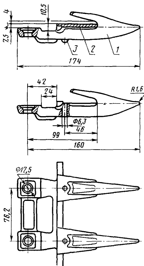
Тип 2 Исполнение 2
