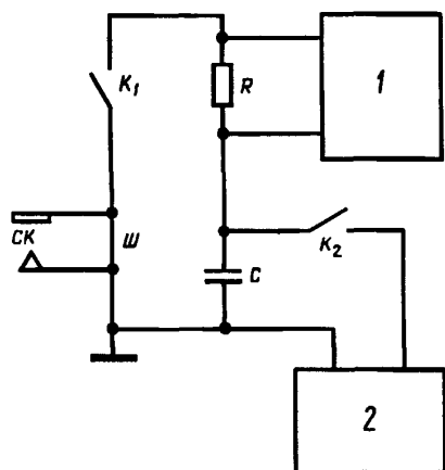
1 — регистратор; 2 — источник питания; R — сопротивление; C — конденсатор; СК — синхроконт- такт; K_1 и K_2 — контакты; Ш — шунт
