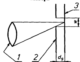
1 — съемочный объектив; 2 — шторка; 3 — фокальная плоскость
