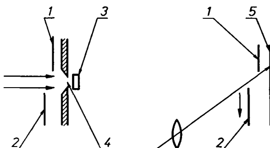
Измерение в параллельном и наклонном световых пучках
