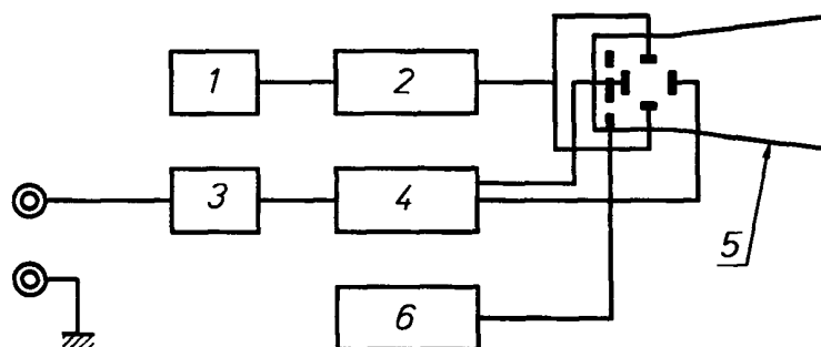
Испытательная схема для апертурных затворов
