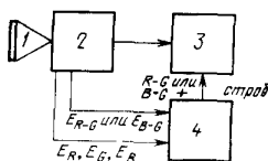
1 — испытательная таблица 3; 2 — камерный канал, 3 — ВКУ по п. 2.1.6; 4 — измеритель совмещения растров по п. 2.1.10
