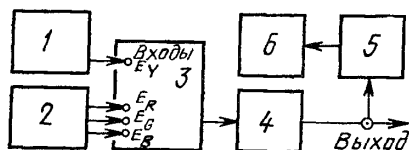
1 — генератор по п 217; 2 — генератор по п 2112; 3 — кодирующее устройство, 4 — последующие блоки канала изображения, 5 — измеритель уровней по п 2113 или 2115 6 — ВКУ по п. 216
