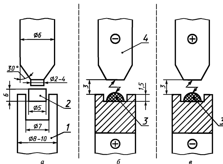
а — расположение и размеры электродов и брикета до экспонирования; б — съемка в анодном режиме; в — съемка в катодном режиме. 1 — графитовая подставка; 2 — брикет; 3 — расплав; 4 — подставной электрод
