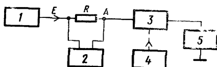
1—источник питания; 2—измеритель постоянного напряжения; 3—микромодуль; 4—генератор; 5—нагрузка; R—резистор.
