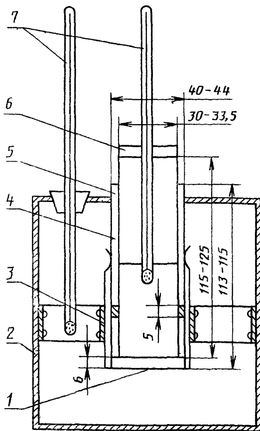
1—диск; 2—баня; 3—прокладка; 4—пробирка; 5—мфта; 6—корковая пробка; 7—термометр
