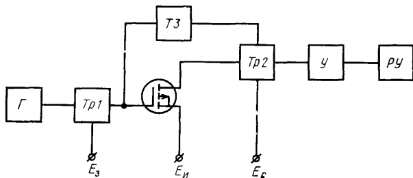
\Gamma —генератор; Тр1 —входной трансформатор полного сопротивления; Тр2 —выходной трансформатор полного сопротивления; Т3 —схема нейтрализации; У —усилитель; РУ —регистрирующее устройство.
