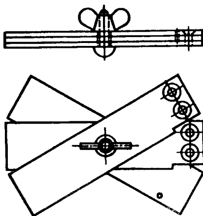
Рисунок 2 — Форма для изготовления цилиндрических образцов золы
