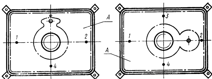
Вид на кинескоп со стороны горловины баллона
