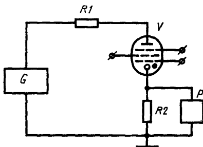
G — источник напряжения; R1 — ограничительный резистор; R2 — измерительный резистор; P — осциллограф; V — испытываемый тиратрон
