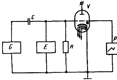
C — переходной конденсатор, E — фильтр, G — источник импульсного напряжения P — осциллограф, R — резистор угетки, V — ис- пытываемый тиатрон
