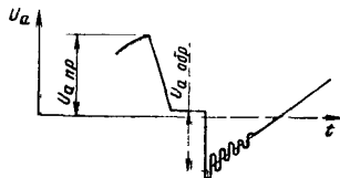
U_{a.пр} — прямое напряжение анода тиристора; U_{a.обр} — обратное напряжение анода тиристора Черт. 20
