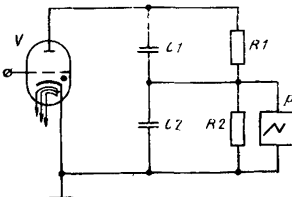
C1, C2 — конденсаторы делителя; P — осциллограф; R1, R2 — резисторы делителя; V — испытываемый тиристор Черт. 19
