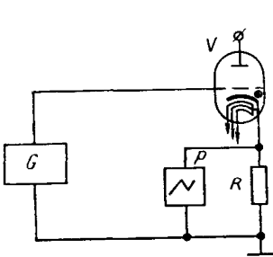
G — источник импульсного напряжения; P — осциллограф; R — измерительный резистор; V — испытываемый тиратрон
