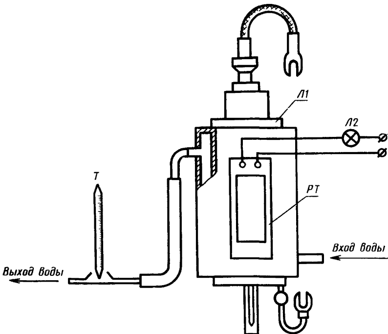
Л1—игнитрон; Л2—сигнальная лампа; РТ—реле тепловой защиты; Т—термометр
