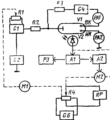
M1 —синхронный двигатель, G1 , G2 , G4 , G6 —стабилизированные источники напряжения с регулируемым выходом, R1 , R4 —линейные потенциометры, R2 , R3 —резисторы, PA1 , PA2 —измерители тока V1 —испытуемый индикатор, V2 —фотодиод, P3 —измеритель сигнала фотодиода, A1 —фотоусилитель, A2 —электронный усилитель, M2 —реверсивный двигатель, RP —электронный самопишущий потенциометр
