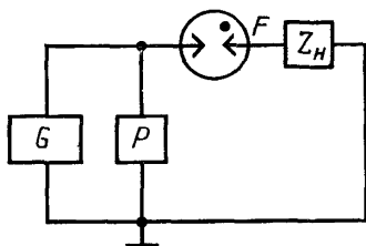
G —источник импульсного напряжения; P —измеритель напряжения; F —испытываемый разрядник; Z_H —нагрузка или эквивалент нагрузки
