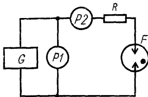
R —защитный резистор; P1 —измеритель напряжения; P2 —измеритель тока; F —испытываемый разрядник; G —источник постоянного напряжения
