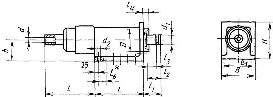
Исполнение 1
