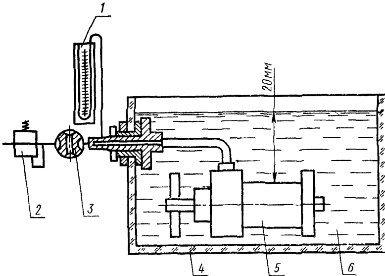
1—манометр по ГОСТ 9933—75, 2—регулятор давления; 3—кран, 4—ванна; 5—испытуемый фильтр, 6—бензин Б-70.
