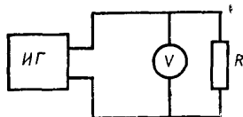
ИГ—генератор импульсов, V— вольтметр, R—испытуемый ре- зистор
