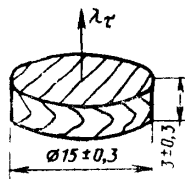
Черт. 3
