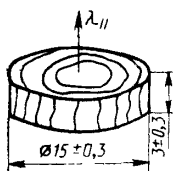
Черт. 1.
