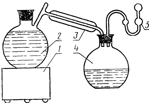
1—электролитка; 2—дистилляционная колба; 3—холодильник; 4—колба-приемник; 5—предохранительная воронка
