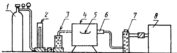
Рисунок 1 — Установка для определения углерода
