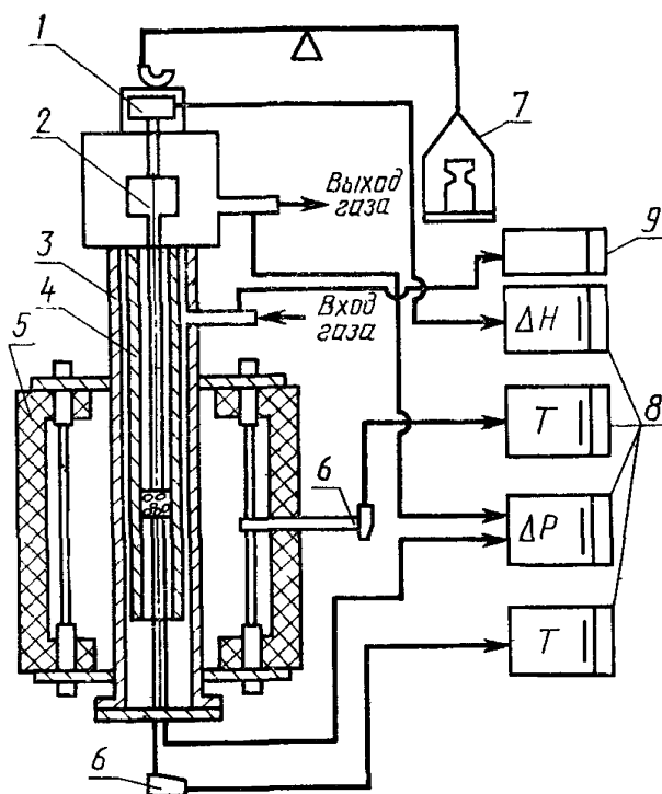
1—датчик для регистрации высоты слоя; 2—шток с грузом; 3—внешняя стенка реакционной камеры; 4—внутренняя стенка реакционной камеры; 5—электродпечь; 6—термопары; 7—взвешивающее устройство; 8—контрольно-измерительные приборы; 9—регулятор подачи восстановительного газа
