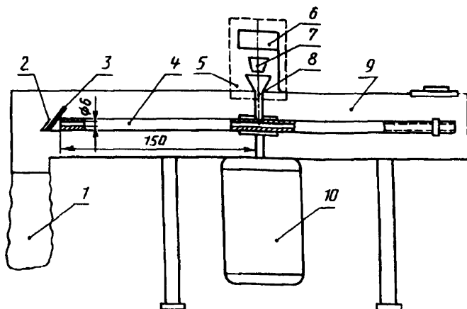
Рисунок 1 — Центробежный абразивметр
