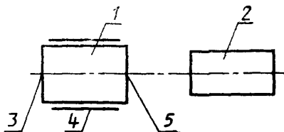
1—ЭОП; 2—яркомер; 3—фотокатод; 4—держатель; 5—экран
