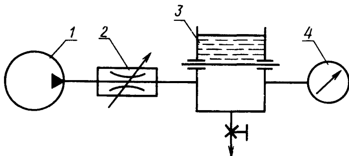
Установка для определения герметичности
