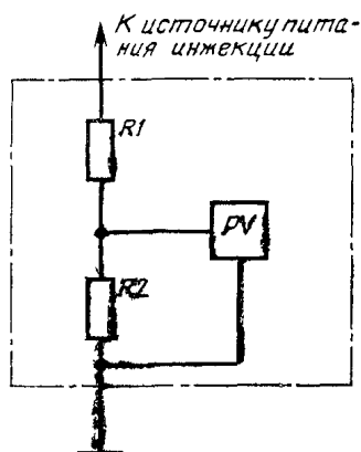
R1, R2 — резисторы делителя; PV — импульсный вольтметр
