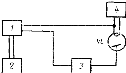
1 — управляемый источник напряжения свыше 1000 В, 2 — устройство задания длительности прохождения тока рентгеновской трубки, 3 — измеритель количества электричества, 4 — источник питания накала, VL — рентгеновская трубка
