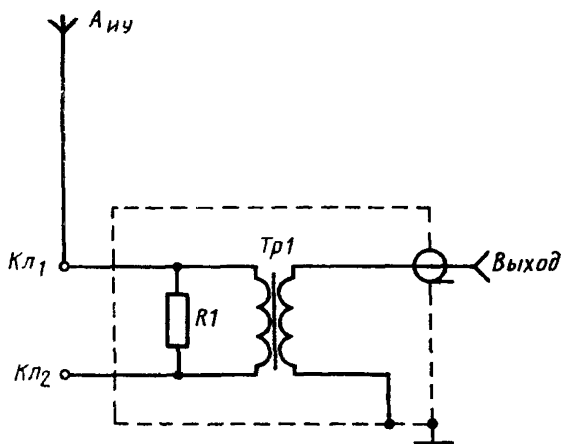
R1 — резистор сопротивлением (10 \pm 1) Ом; Tr1 — трансформатор (черт. 3); KЛ1 — зажим для присоединения антенны A_{ny} ; KЛ2 — зажим для присоединения антенны A_n .
