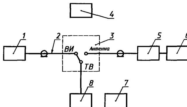
1 — ВИ; 2 — соединительный кабель, входящий в комплект ВИ; 3 — антенный переключатель, входящий в комплект ВИ; 4 — генератор замещающих сигналов; 5 — согласующий аттенюатор; 6 — измеритель радиопомех; 7 — контрольный ТВ (монитор); 8 — эквивалент нагрузки сопротивлением 75 Ом
