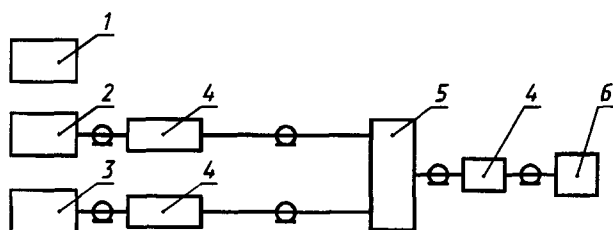
1 — генератор замещающих сигналов; 2 — испытуемое устройство; 3 — генератор испытательных сигналов; 4 — согласующий аттенюатор; 5 — разветвитель; 6 — измеритель радиопомех
