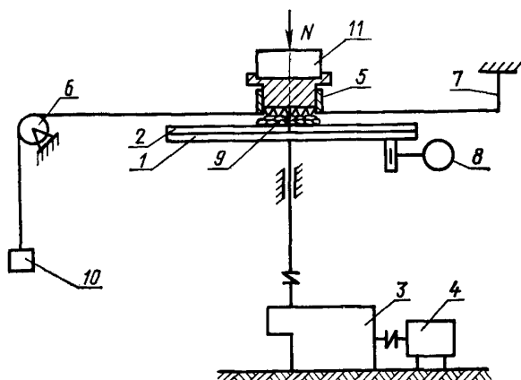
Схема испытаний и тарировки
