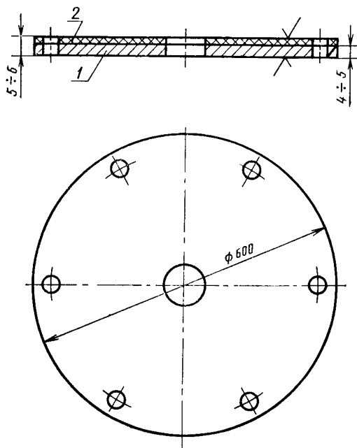
Образец исследуемого материала
