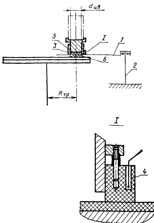
I — стрела; 2 — вертикальная ось; 3 — цилиндрический короб; 4 — скользящий элемент (медный электрод); 5 — поршень; 6 — волокнистая масса
