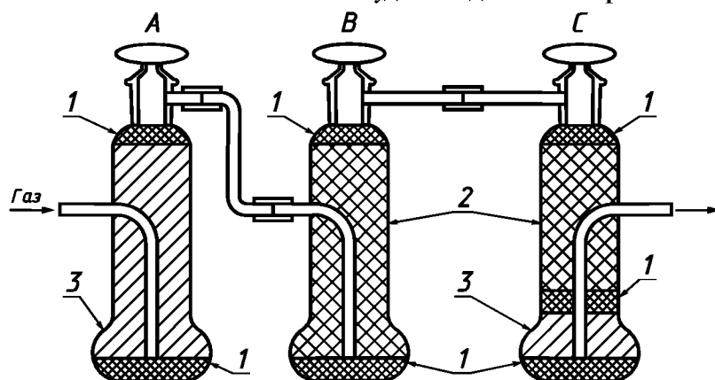
А — сосуд для поглощения воды; В и С — сосуды для поглощения диоксида углерода 1 — стекловата (или вата гигроскопическая); 2 — гидроксид натрия на инертной основе (аскарит); 3 — перхлорат магния (ангидрон)
