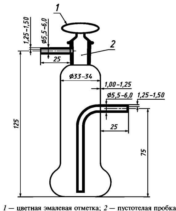
Рисунок 2 — Сосуд Мидвэйла
