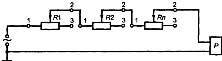
R_1, R_2, \dots, R_n — проверяемые резисторы; 1, 2, 3 — выводы проверяемых резисторов; P — осциллограф
