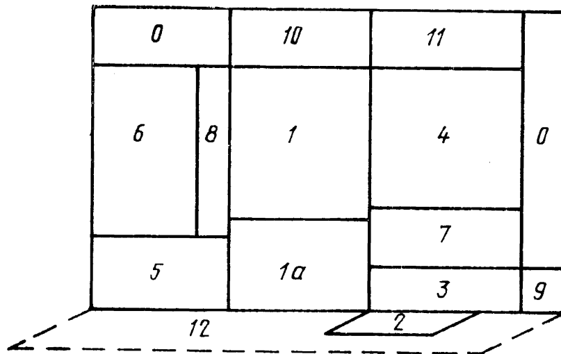
Взаимное размещение зон на приборной доске бортинженера
