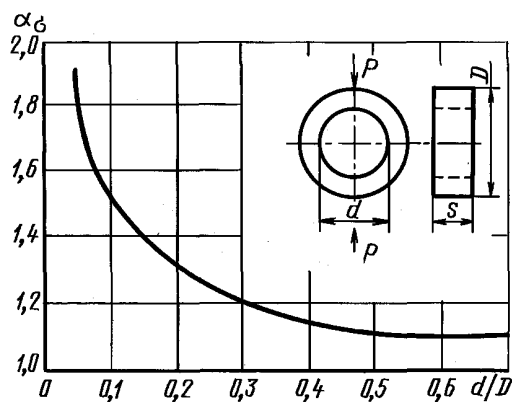
Кольцо с наружной единичной нагрузкой P
