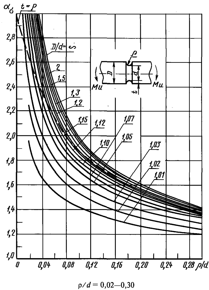
Валы с выточкой при изгибе (черт. 14—16)
