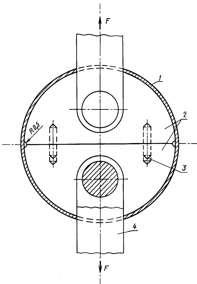
1 — образец; 2 — полудиски; 3 — направляющая; 4 — тяга
