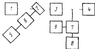
1—источник импульсов оптического излучения на основе лазера; 2—делительная пластина; 3, 6—измерительные ослабители; 4—СИ ММ с известными параметрами; 5—контрольное средство измерений; 7—камера с исследуемым фотоэлементом; 8—источник питания фотоэлемента; 9—импульсный вольтметр или осциллограф
