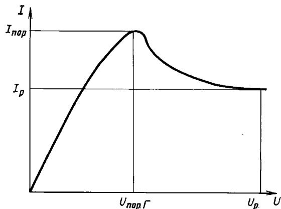
Вольт-амперная характеристика диода Ганна
