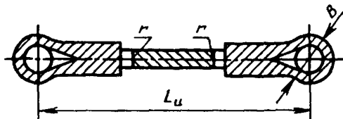
Машина для испытаний с кнехтами для наросенных петель (отметка r расположена на расстоянии 150 мм от последнего витка сращивания)
